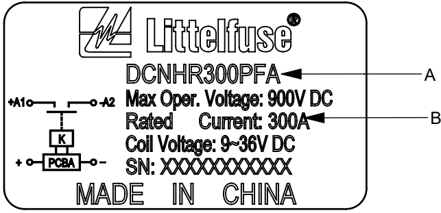
SCALE 2:1
