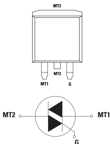
TO-263
