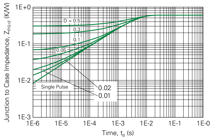
Fig. 25. Thermal Impedance
