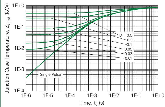
Fig. 25. Thermal Impedance
