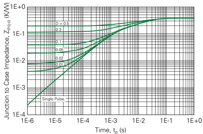
Fig. 25. Thermal Impedance
