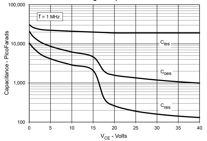
Fig. 8. Capacitance
