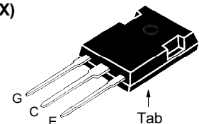
PLUS247 (IXGX)
