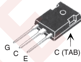
TO-247 (IXGH)
