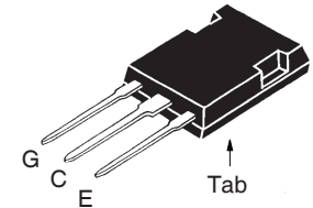
PLUS247™ (IXGX)
