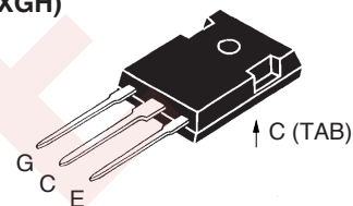
TO-268 (IXGT)
