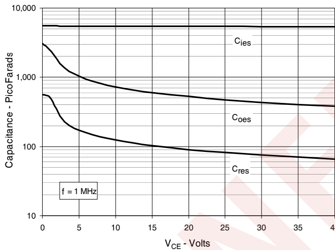
Fig. 9. Capacitance
