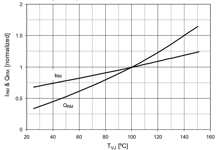
Fig. 26. Dynamic Parameters Q_{RM} , I_{RM} vs. T_{VJ}
