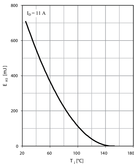
Fig. 10 Avalanche energy
