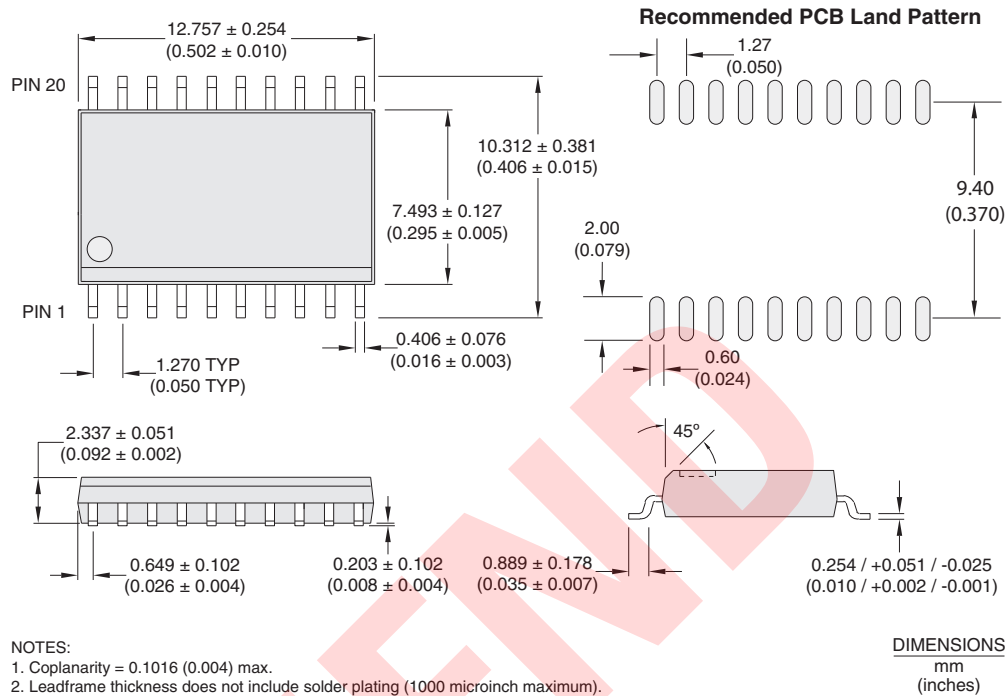
CPC7695Zx Package
