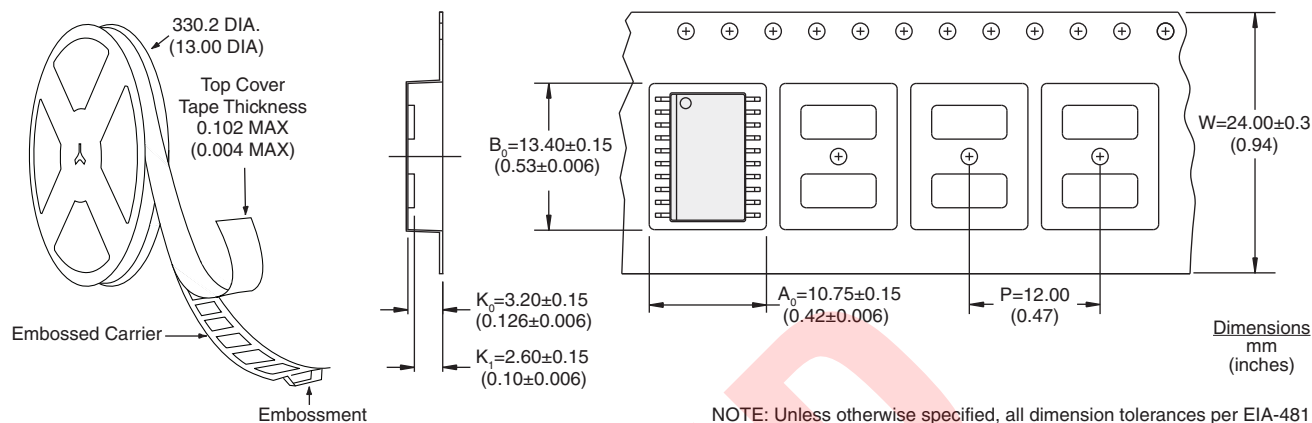
CPC7695ZxTR Tape &amp; Reel
