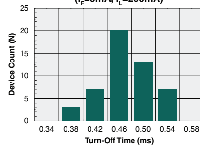
Turn-Off Time Distribution ( I_F=5\text{mA} , I_L=200\text{mA} )
