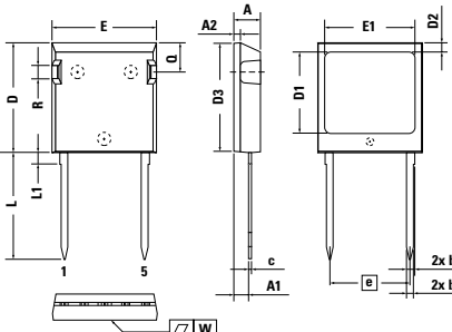
X024e ISOPLUS i4-PAC™ Weight = 6 g
