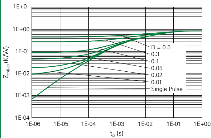
Fig. 7. Transient Thermal Impedance
