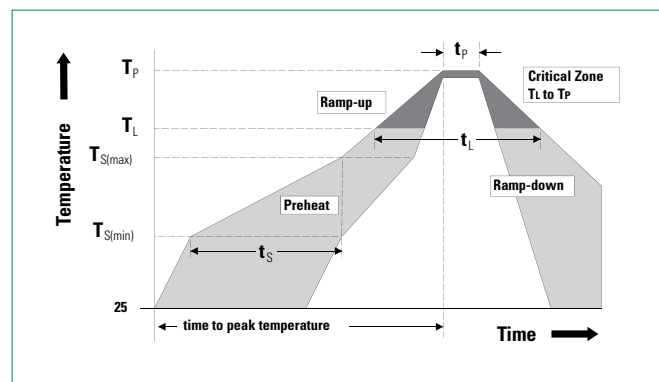
Soldering Parameters
