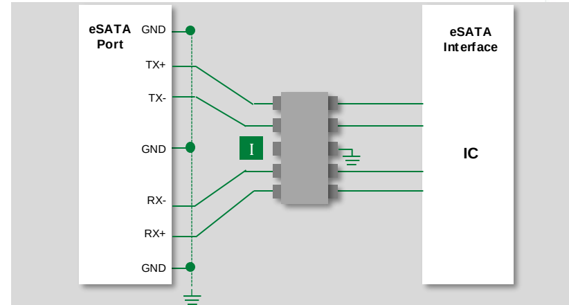
eSATA
