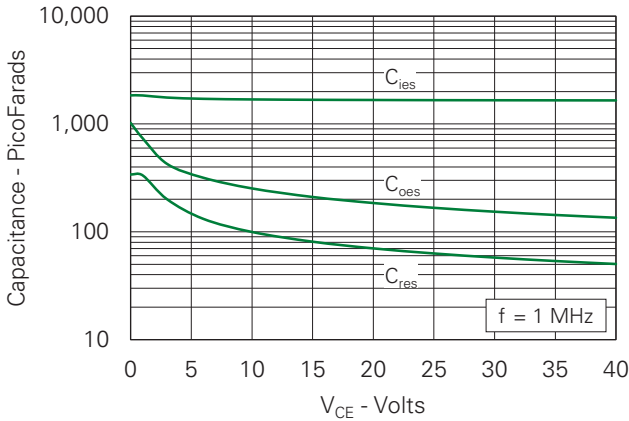
Fig. 9. Capacitance
