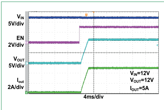
EN Power On
