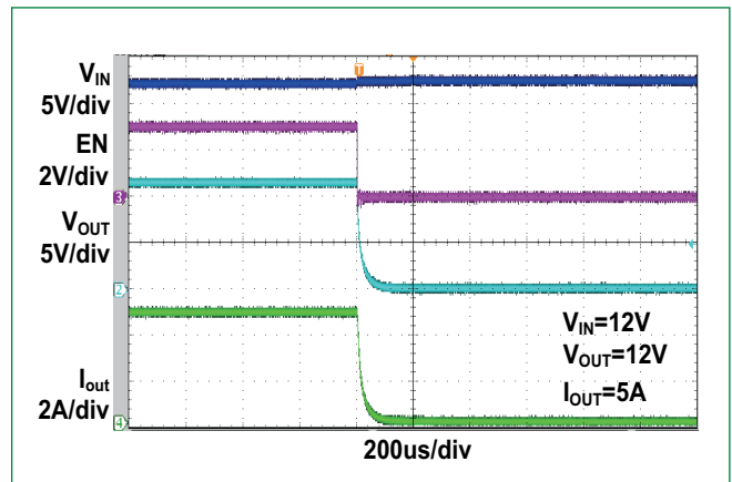
EN Power Off
