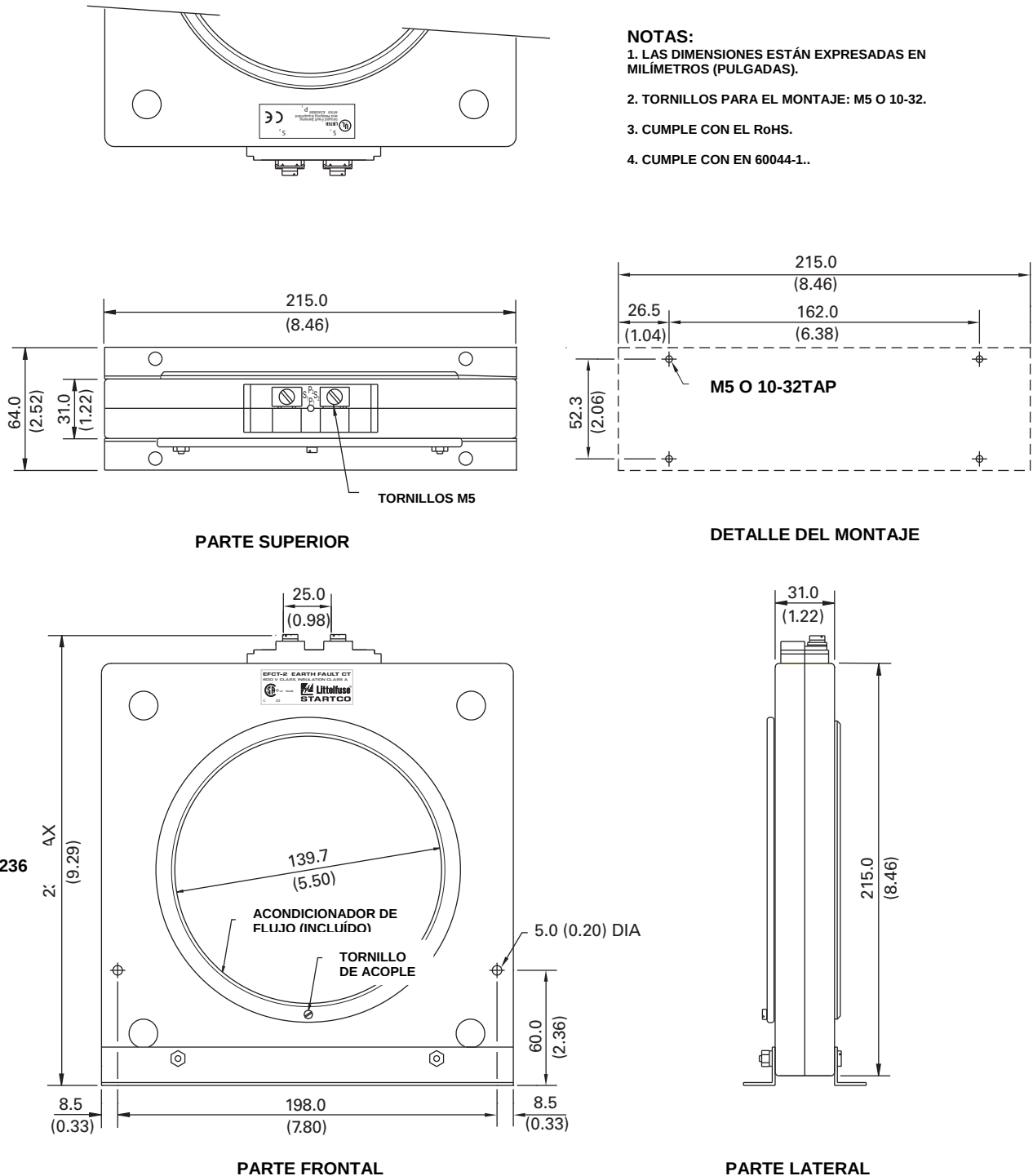
FIGURA 8. Esquema y detalles de montaje del EFCT-2
