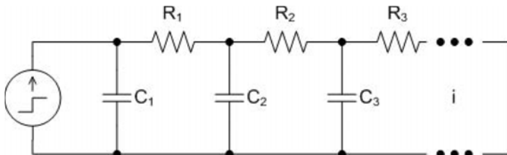
Fig. 22. Cauer Thermal Network
